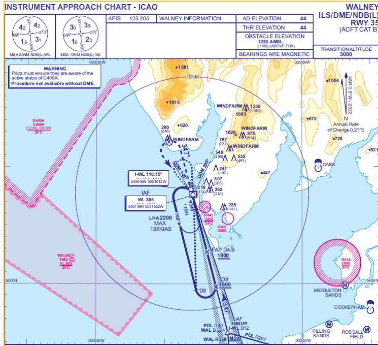
Figure 224 - ILS/DME/NDB(L) RWY 35
