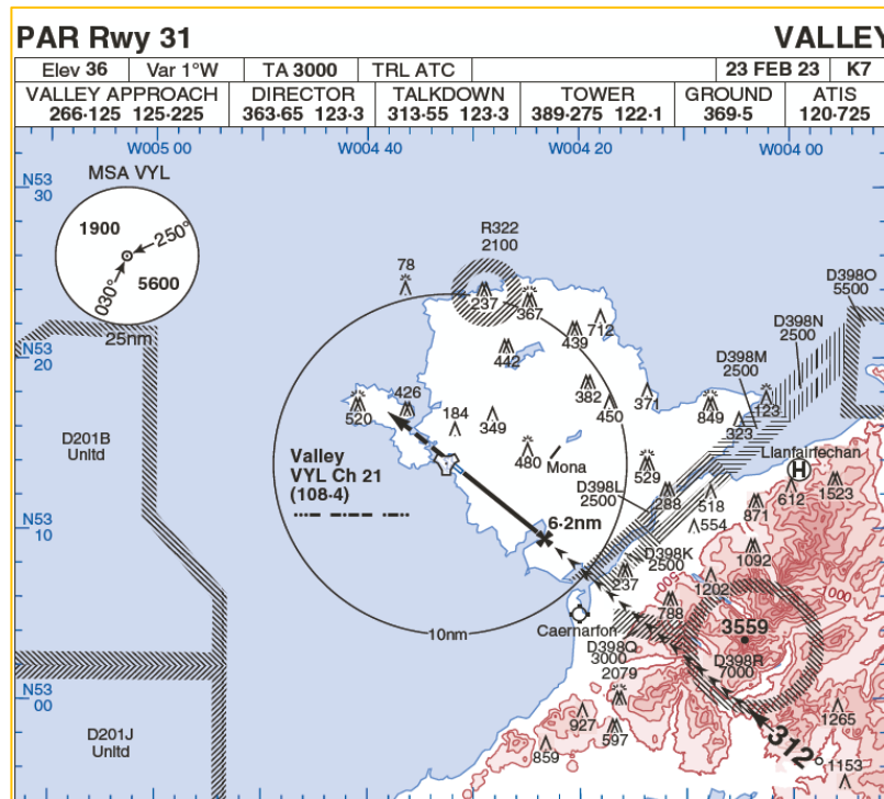
Figure 171 - PAR RWY 31 Procedure
